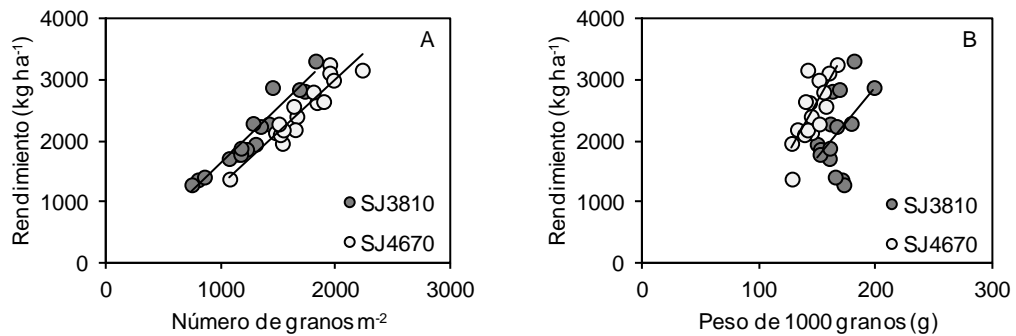
Figura 22. Rendimiento en función del: A. Número de granos m -2 . B. Peso de mil granos, de 16 unidades observacionales de los tratamientos SJ3810 y SJ4670.
