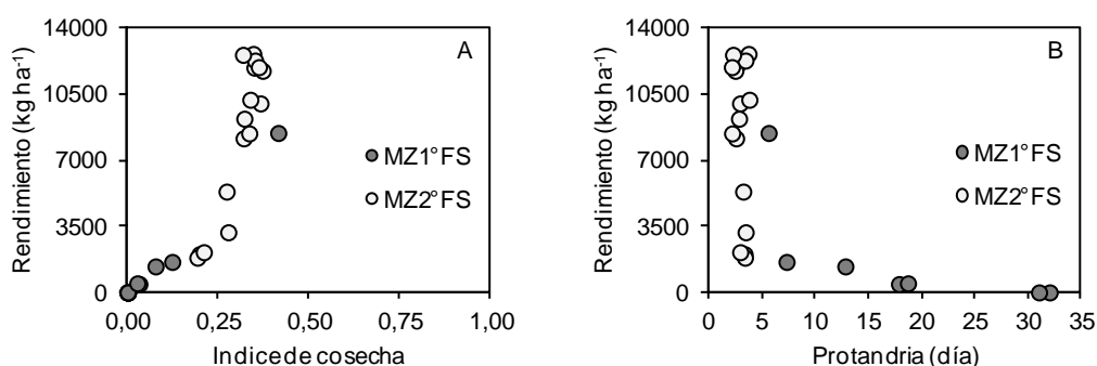
Figura 16. Rendimiento en función de: A. Índice de cosecha. B. Protandria, de 16 unidades observacionales de los tratamientos MZ1°FS y MZ2°FS. MZ1°FS: cultivos de maíz de fecha de siembra temprana (03/10/2011). MZ2°FS: cultivos de maíz de fecha de siembra tardía (13/12/2011).
