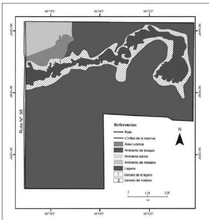
Figura 2. Delimitación de los ambientes del Parque Luro.
