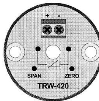
Conexión 2 hilos
