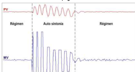
Figura 11 – Ejemplo de una auto sintonía
