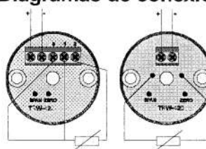
Conexión 3 hilos Conexión 2 hilos
