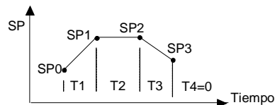
Figura 9 - Ejemplo de programa con pocos segmentos
