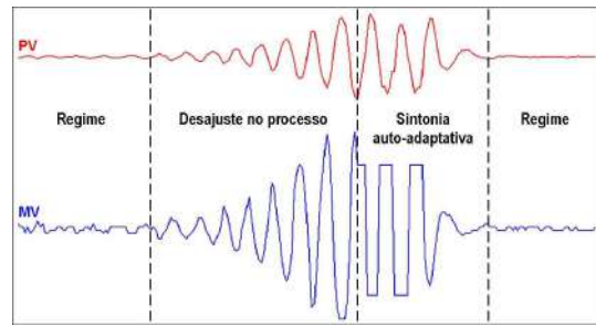
Figura 12 – Ejemplo de una sintonía auto-adaptativa
