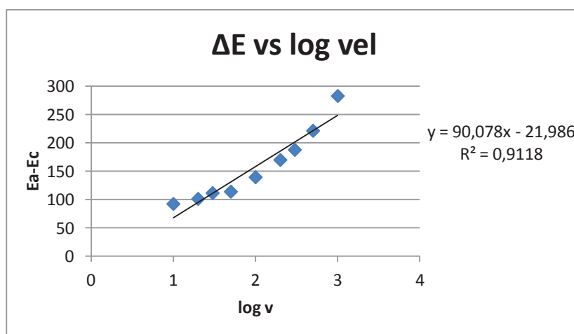
Figura 5.3 Dependencia de la diferencia de potencial ( \Delta E ) entre el potencial del pico anódico ( E_a ) y el potencial del pico catódico ( E_c ), con la velocidad de barrido de potencial, para BNZ (3,9mM) en DMSO. Medio neutro.
